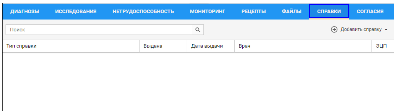
Рисунок 6 – Раздел "Справки"
